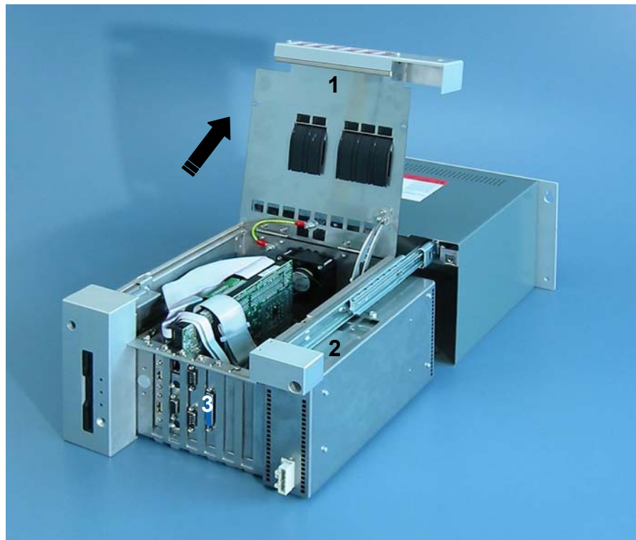
Ansicht des geöffneten PCs
