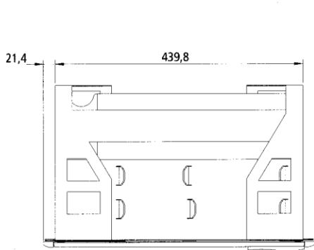
Draufsicht mit Auszugrahmen für Frontmontage
