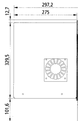
Seitenansicht mit Auszugrahmen für Frontmontage
