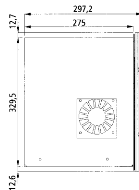
Seitenansicht mit Auszugrahmen für Frontmontage
