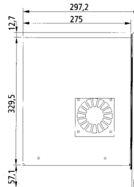
Seitenansicht mit Auszugrahmen für Frontmontage
