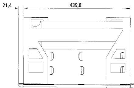
Draufsicht mit Auszugrahmen für Frontmontage
