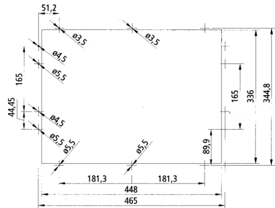
Zum Einbau benötigter Ausschnitt
