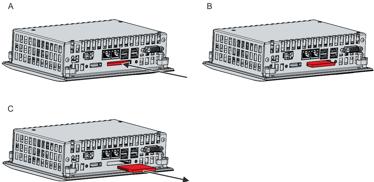
Abb. 23: Austausch CFast
