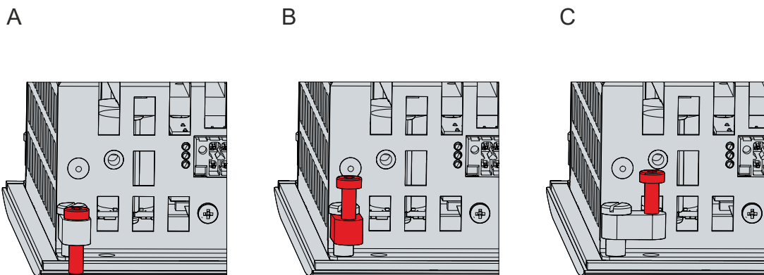
Abb. 18: Demontage aus dem Schaltschrank
