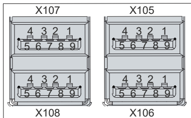
Abb. 6: USB-Schnittstelle Pin-Nummerierung
