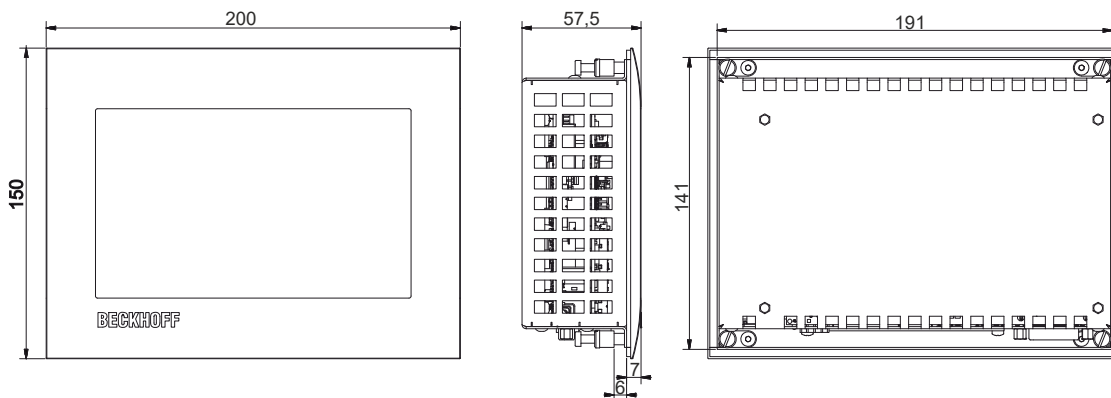
Abb. 10: Abmessungen
