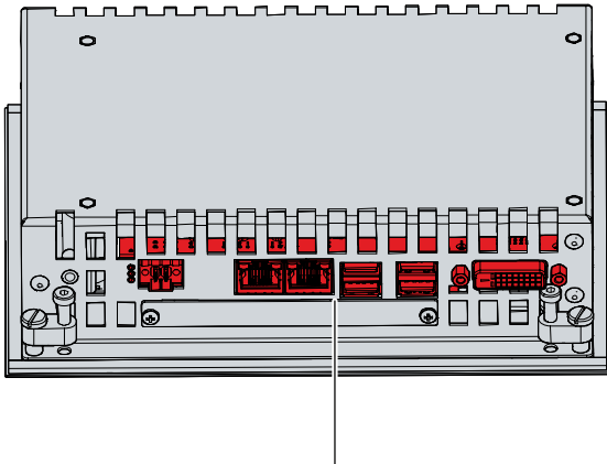
Abb. 3: Anschlussbereich
