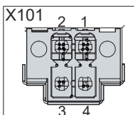
Abb. 4: Spannungsbuchse Pin-Nummerierung
