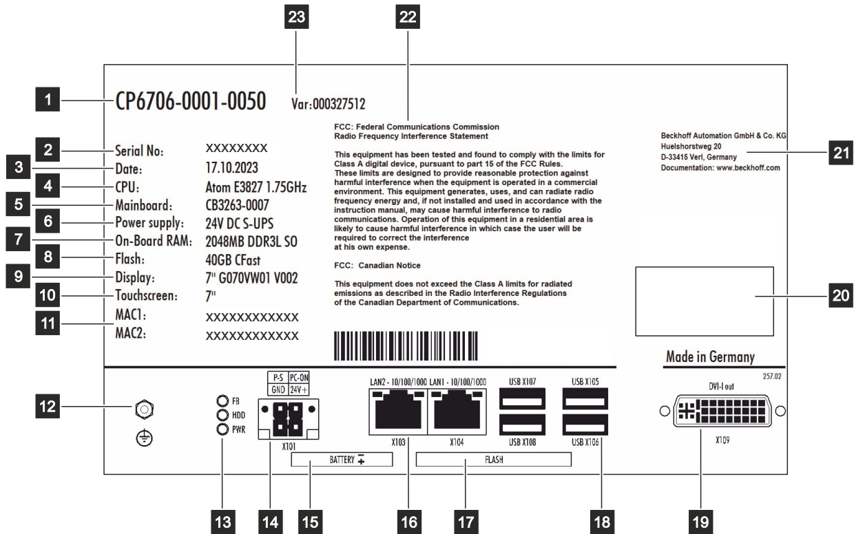
Abb. 9: Typenschild
