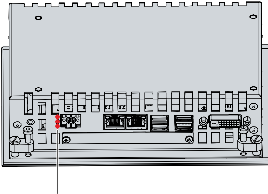
Abb. 8: Status-LEDs
