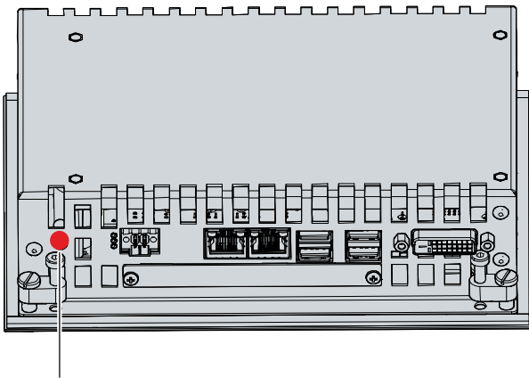
Abb. 15: Schutzleiteranschluss PE
