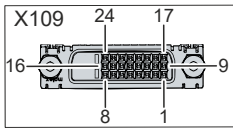
Abb. 7: DVI-Schnittstelle Pin-Nummerierung
