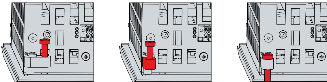
Abb. 14: Schaltschrankeinbau
