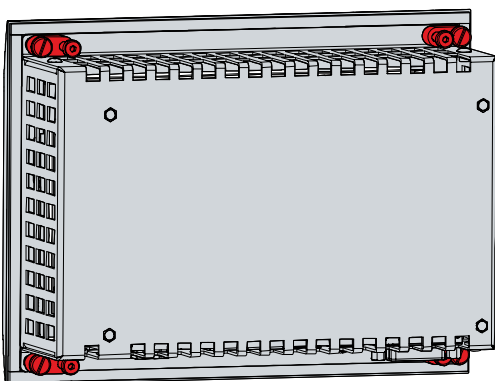
Abb. 12: Auslieferungszustand Klemmhebel
