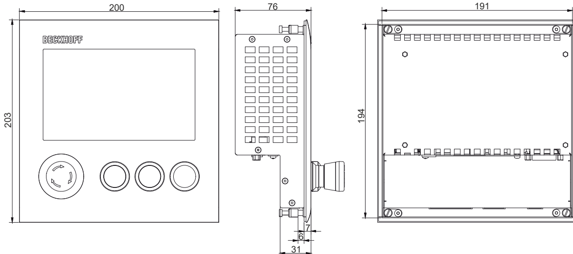
Abb. 11: Abmessungen Tastererweiterung
