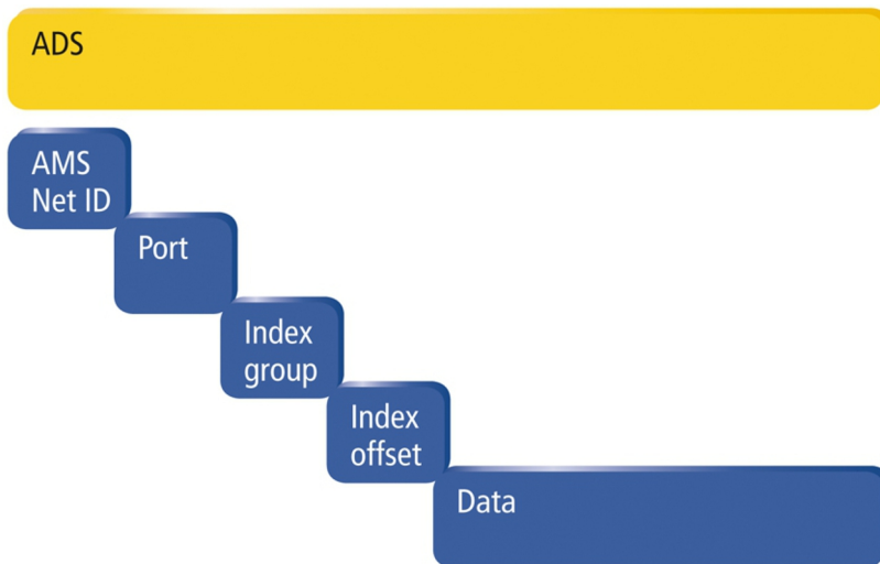
Abb. 15: Aufbau der ADS-Kommunikation.
