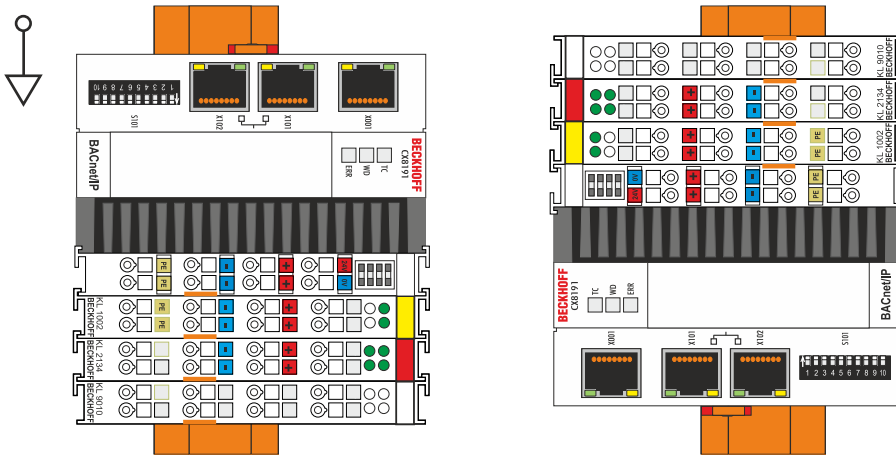
Abb. 6: Embedded-PC CX8191, senkrechte Einbaulage.
