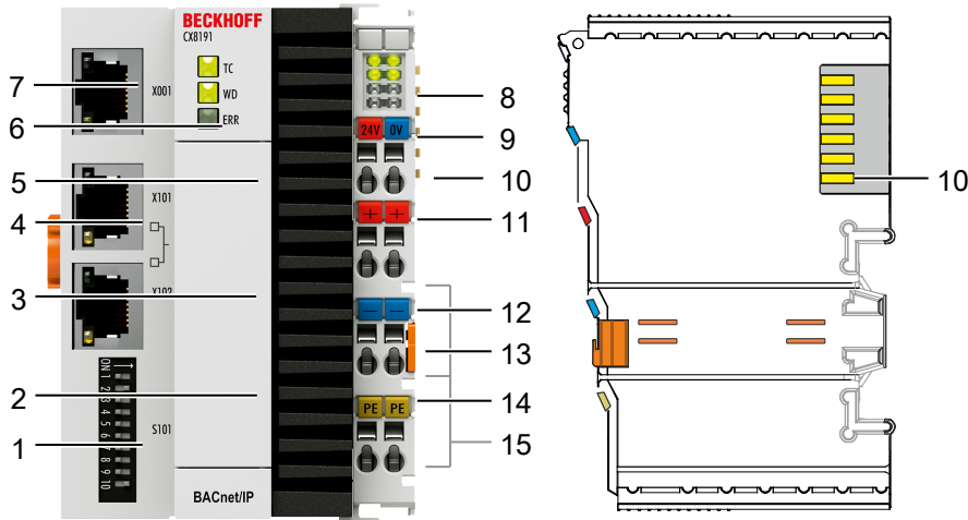
Abb. 1: Beispielaufbau eines Embedded-PCs CX8191.
