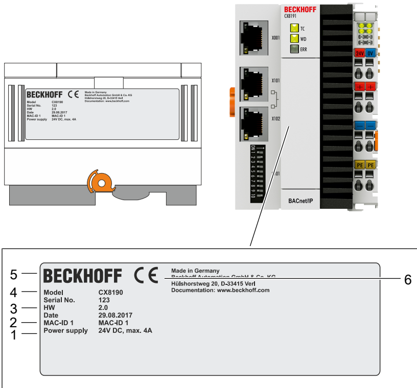
Abb. 2: CX8191 Typenschild.
