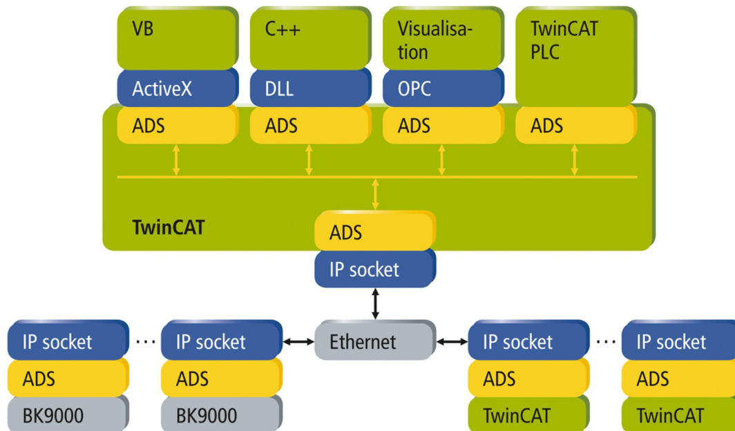
Abb. 14: ADS-Protokoll als Transportschicht innerhalb von TwinCAT.
