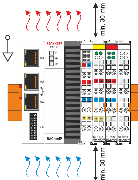
Abb. 5: Embedded-PC CX8191, waagerechte Einbaulage.
