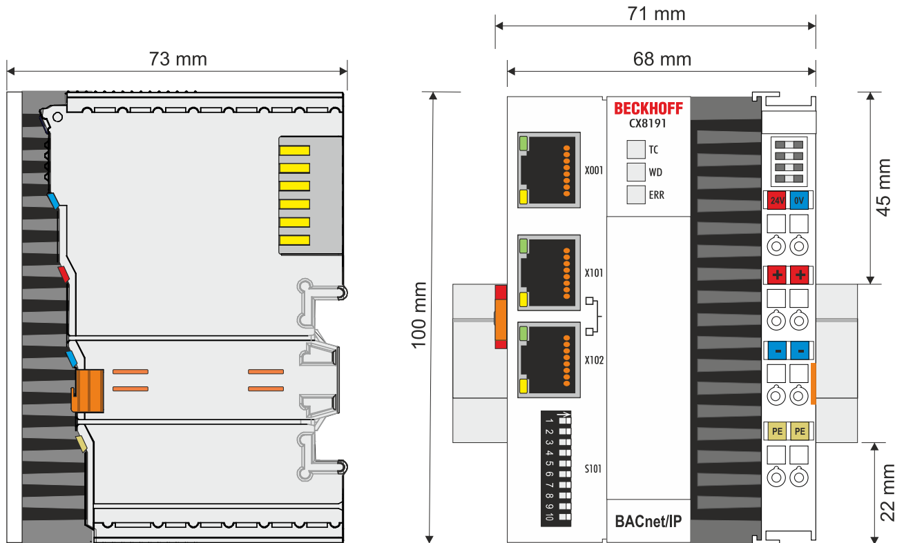
Abb. 4: Abmessungen des Embedded-PCs CX81xx.
