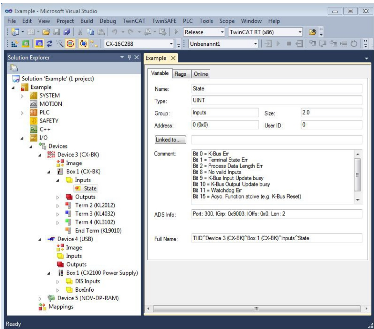
Abb. 16: Status-Variable für Fehlerbehandlung und Diagnose unter TwinCAT.
