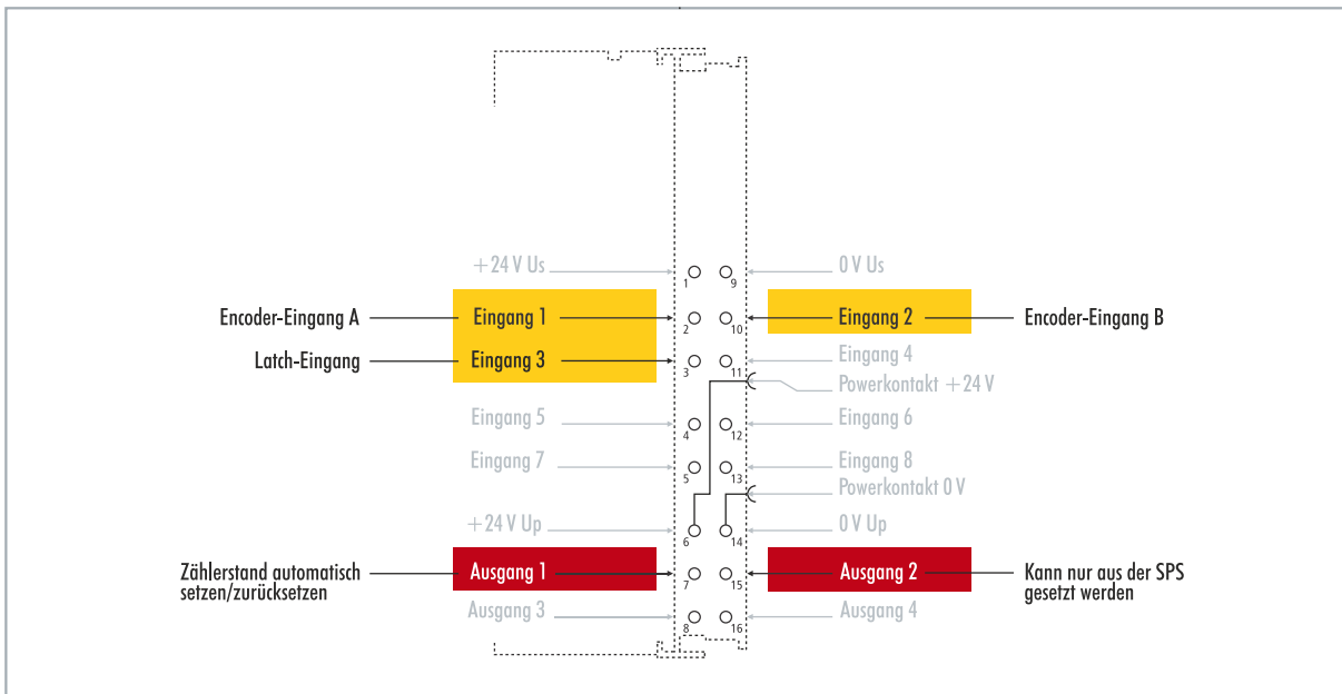
Abb. 20: Konfigurierbare Ein- und Ausgänge im Inkremental-Encoder-Modus.
