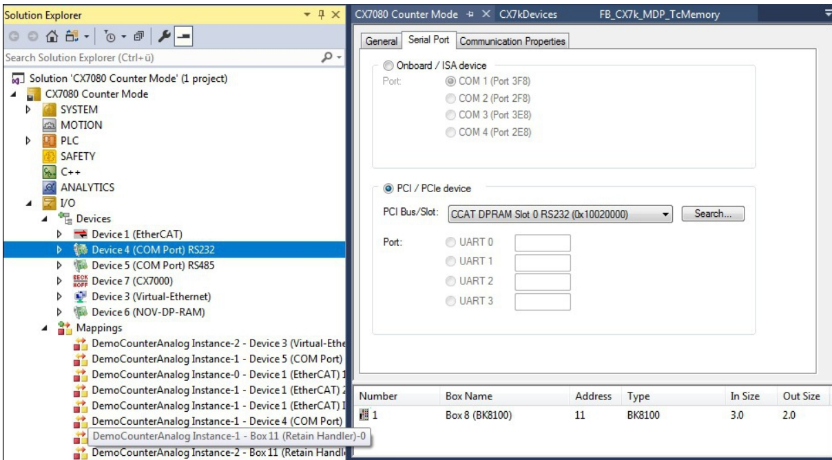
Abb. 26: RS232-Schnittstelle unter TwinCAT 3.
