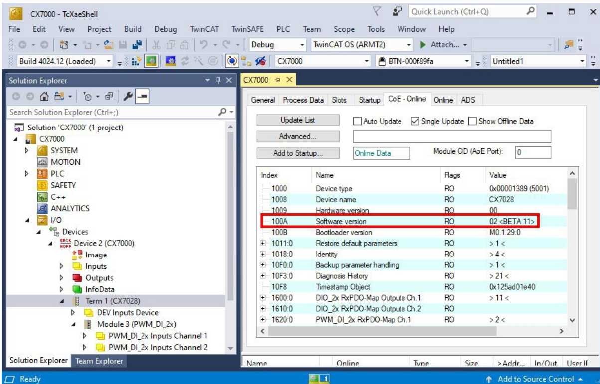
Abb. 30: CoE-Kommunikation, Auflistung der CoE-Objekte mit passender Index-Nummer.
