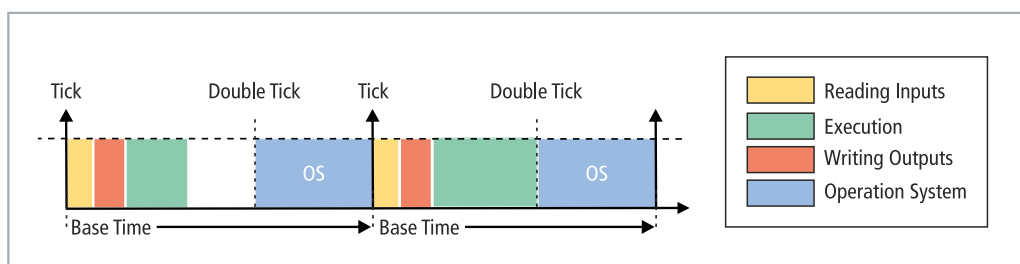
Abb. 39: Aufruf einer SPS-Task mit Attribut TcCallAfterOutputUpdate.
