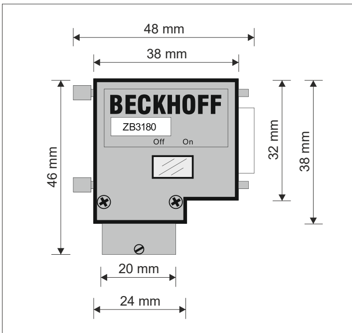
Abb. 53: D-Sub-Stecker ZB3180, Maßzeichnung.
