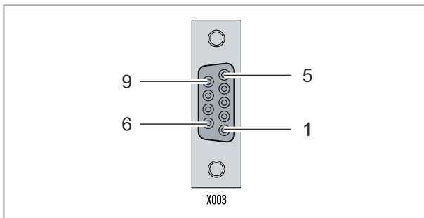
Abb. 4: RS232/RS485-Schittstelle X101
