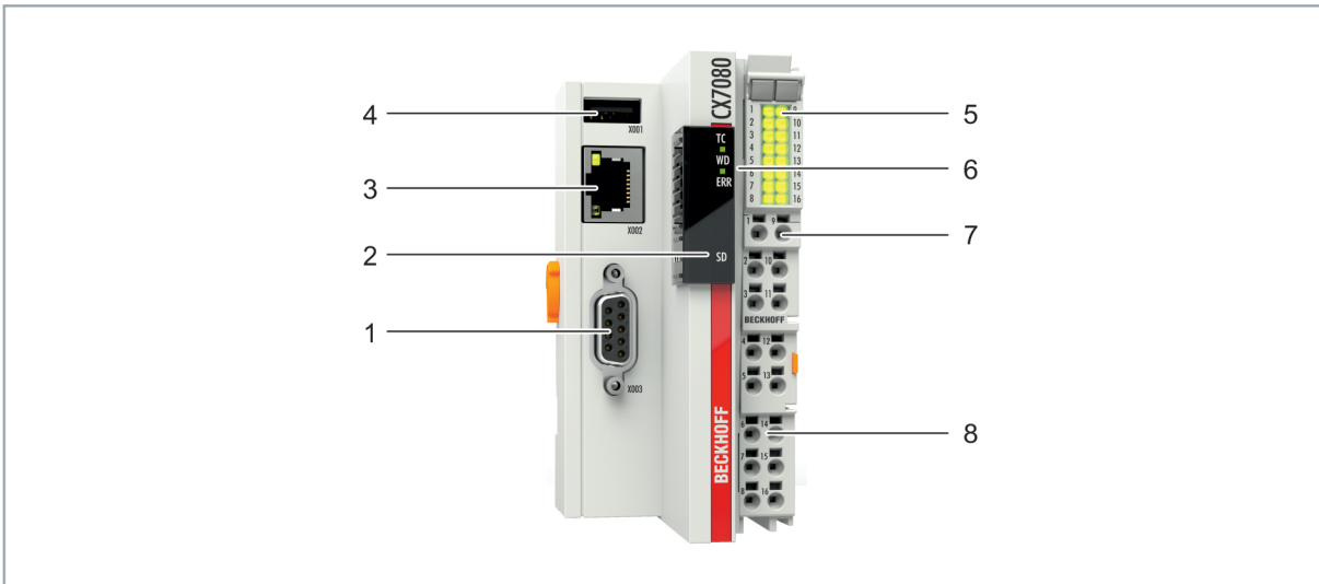
Abb. 1: Beispielaufbau eines Embedded-PCs CX7080.
