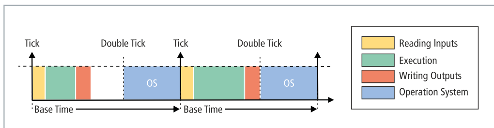
Abb. 38: Standard-Aufruf einer SPS-Task.
