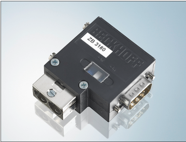
Abb. 52: D-Sub-Stecker ZB3180 mit zuschaltbarem Abschlusswiderstand.
