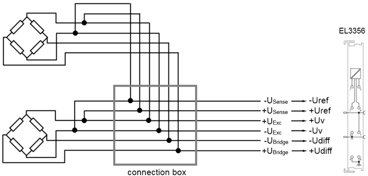
附图 22：并联应变计
