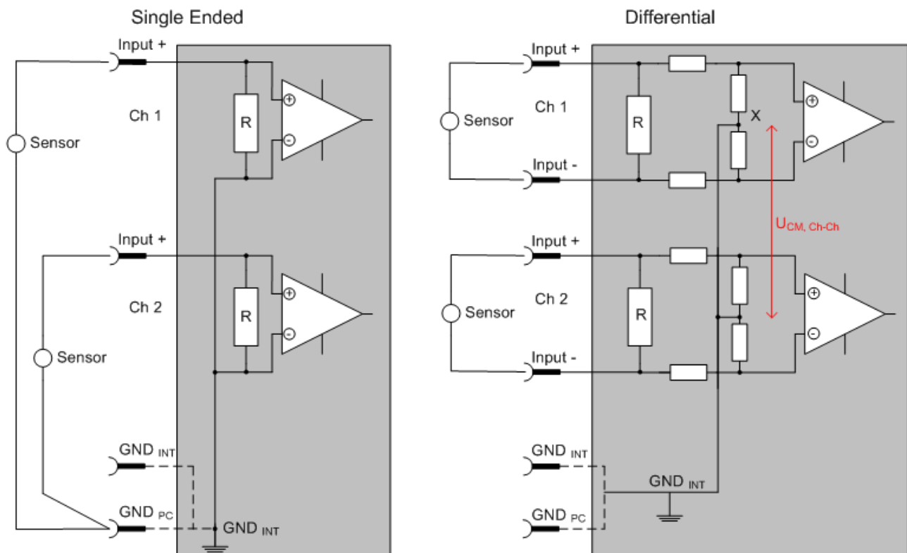
附图 32: SE 和 DIFF 模块为 2 通道版本
