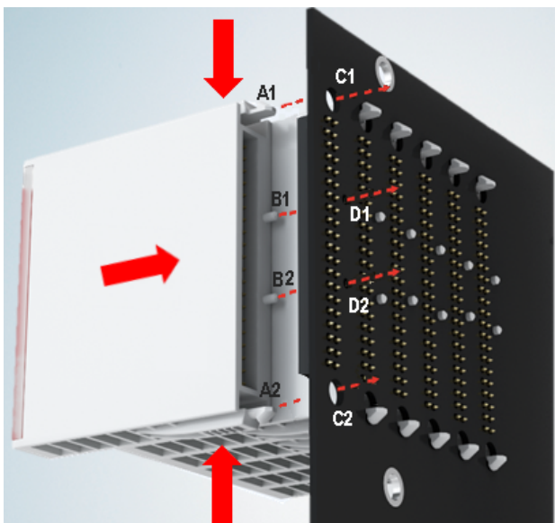
Abb. 19: Montage EJ-Module
