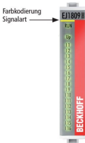
Abb. 16: EJ-Module Farbcodierung am Beispiel EJ1809
