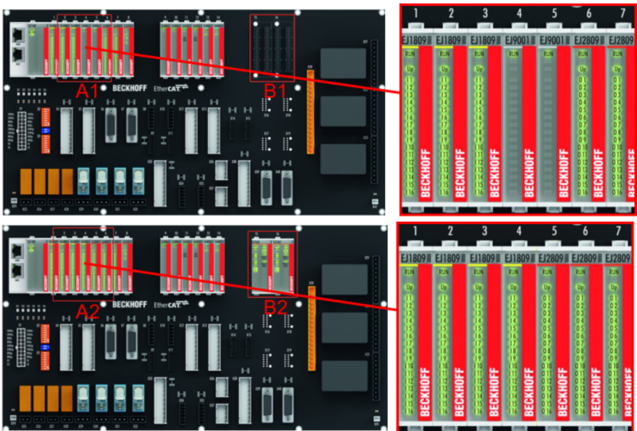
Abb. 20: Beispiel Austausch Platzhaltermodule u. Belegung Reserveslots
