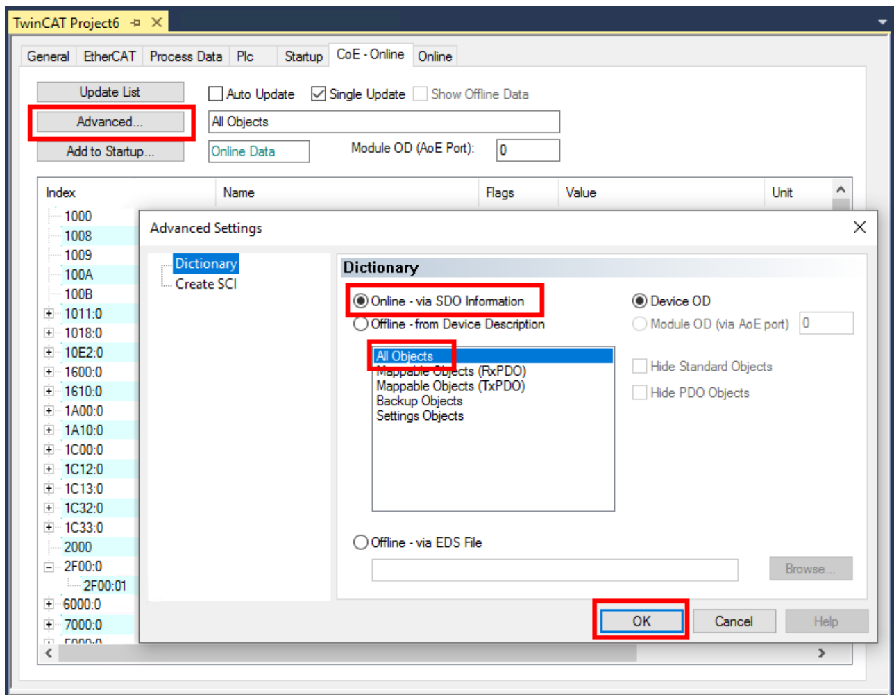
Abb. 37: Vollständiger Reload des CoE-Verzeichnisses
