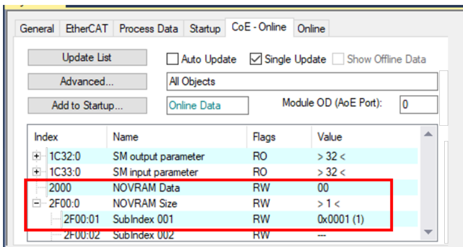
Abb. 33: Beliebiger Startzustand des Moduls EJ6080
