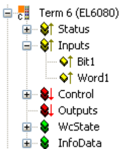
Abb. 31: Unzulässige Konfiguration am Beispiel EL6080 bis TwinCAT b2.10 b1330
