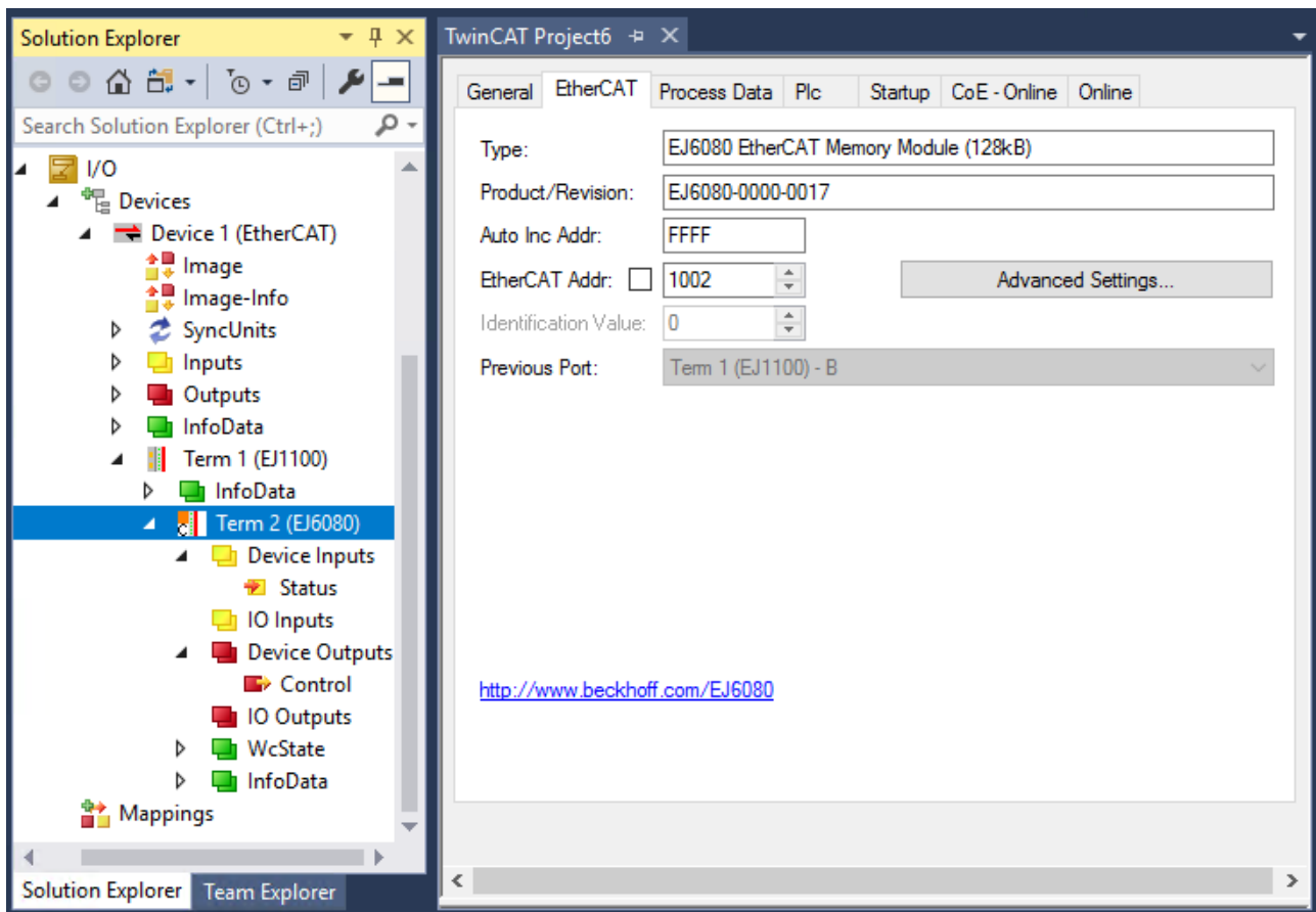
Abb. 26: Default Prozessabbild der EJ6080 nach dem Einfügen
