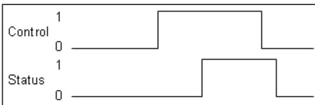
Abb. 32: Zyklischer Betrieb mit Handshake
