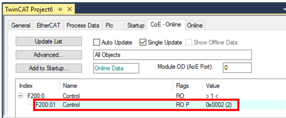
Abb. 39: Lock im CoE
