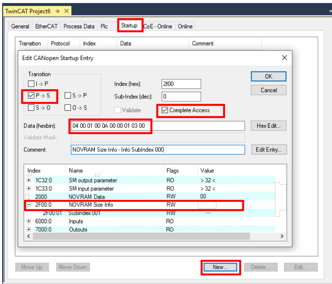
Abb. 34: Definition eines neuen StartUP-Eintrags
