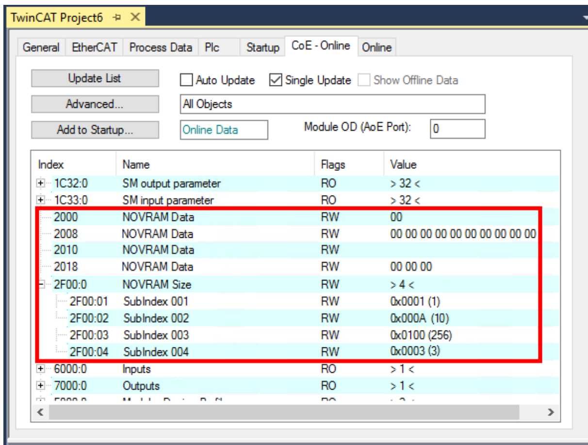
Abb. 38: Geändertes CoE-Verzeichnis
