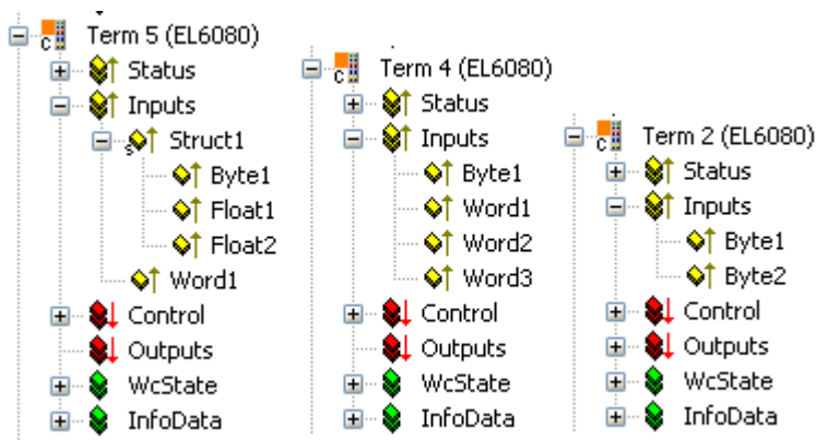
Abb. 30: Zulässige Konfiguration am Beispiel EL6080
