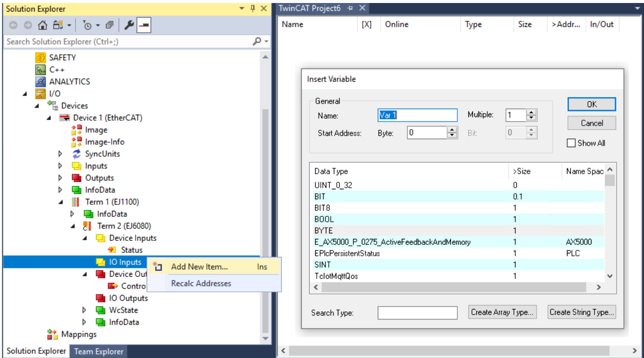
Abb. 29: Manuelles Anlegen der zyklischen Prozessdaten
