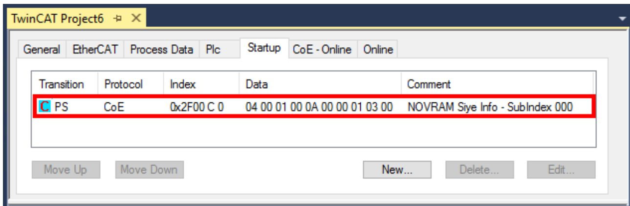
Abb. 35: Neuer StartUp-Eintrag
