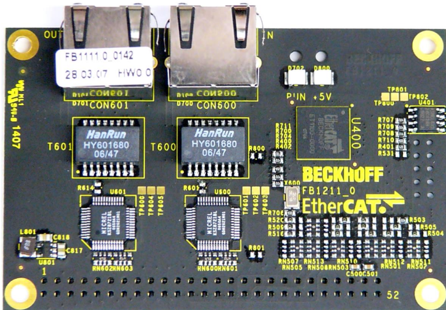
Abbildung 2 Feldbusbriefmarke FB1111-0142
