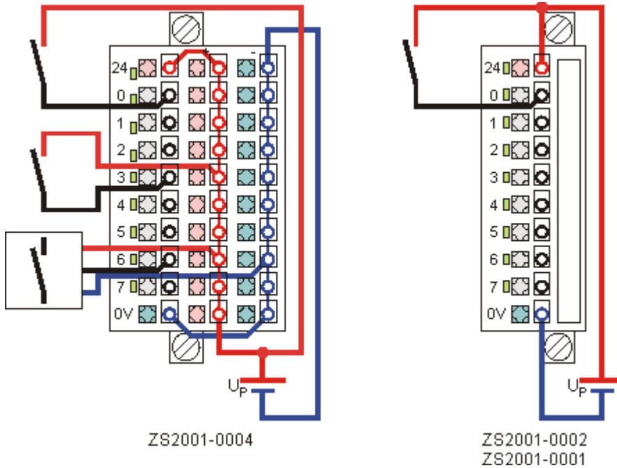
Abb. 18: Anschluss
