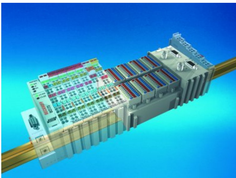
Abb. 1: Busklemmenblock
