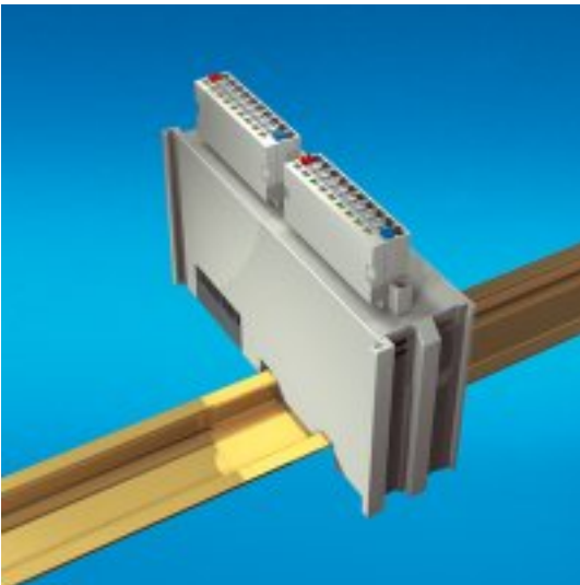
Abb. 3: Klemmenmodul mit Steckverbinder für Einleiteranschlussstechnik (ZS2001-0002)
