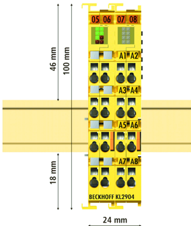
Abb. 5: Abmessungen
