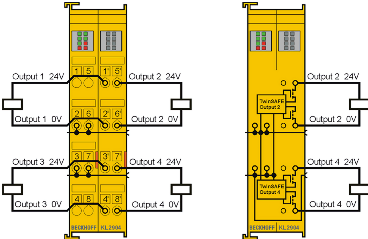
Abb. 10: Anschlussbelegung der KL2904
