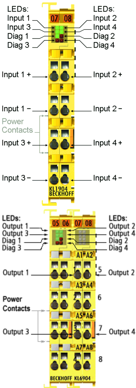
Abb. 3: TwinSAFE-Klemmen (EtherCAT)
