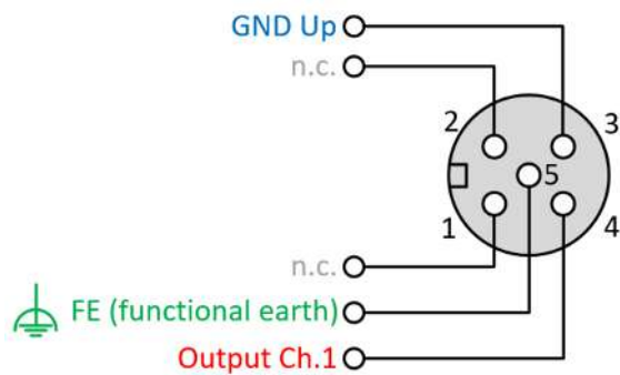
Abb. 10: PinOut sicherer Ausgang
