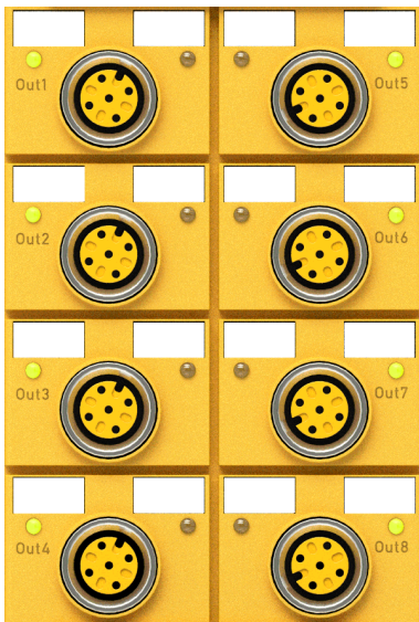
Abb. 9: Sichere Ausgänge 1 bis 8
