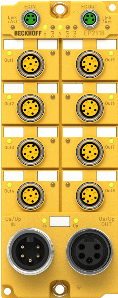
Abb. 26: EP2918 - Status-LEDs
