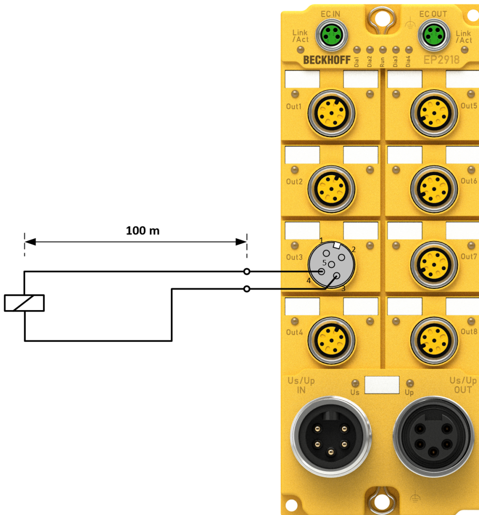
Abb. 11: Signalleitungen
