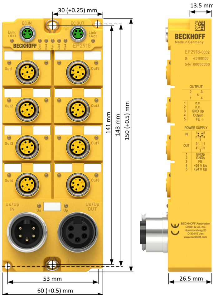
Abb. 3: Abmessungen
