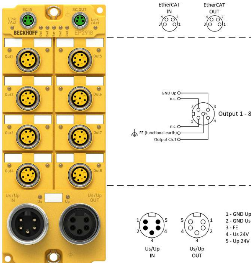
Abb. 2: EP2918 - TwinSAFE-EtherCAT-Box mit 8 fehlersicheren Ausgängen
