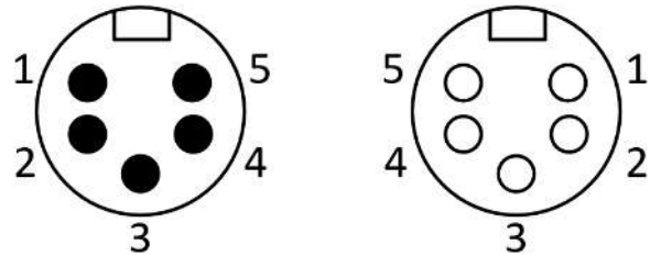
7/8" - Steckerbelegung
